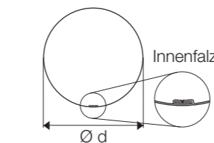
Dachablaufrohre nach EN 612 Abmessungen
