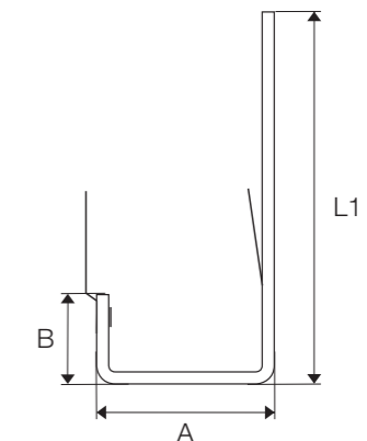
Vierkant-Hängerinnenhaken nach EN 612 Abmessungen
