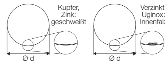
Dachablaufrohre nach EN 612 Abmessungen
