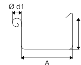
Vierkant-Hängerinnen nach EN 612 Abmessungen
