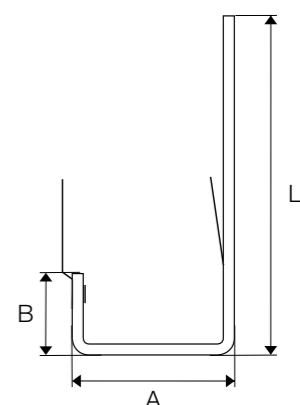
Vierkant-Hängerinnenhaken nach EN 612 Abmessungen
